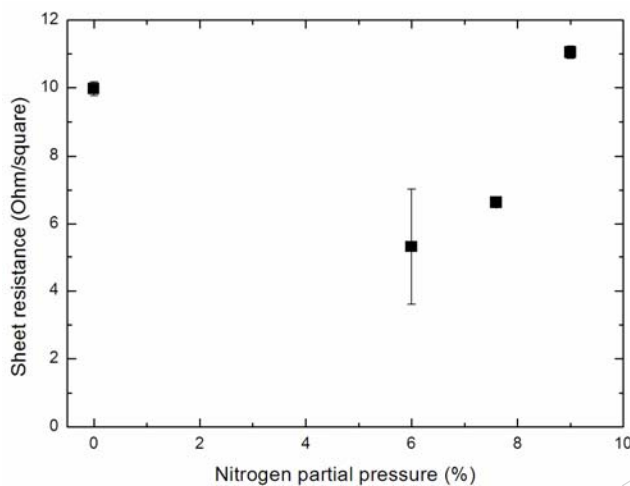
ภาพที่ 3 ความสัมพันธ์ระหว่างความต้านทานแผ่นกับความดันย่อยของแก๊สไนโตรเจน
