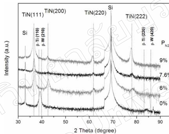
ภาพที่ 1 แบบอย่างการเลี้ยวเบนของฟิล์มไทเทเนียมทั้งสแตนไนไตรด์ที่เคลือบลงบนซิลิกอนระนาบ (100) ที่เปลี่ยนความดันย่อยของแก๊สไนโตรเจน
