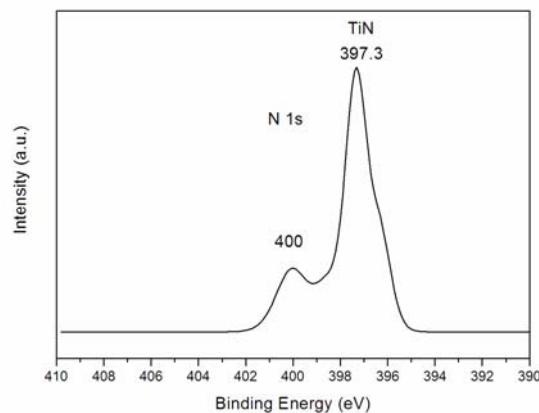
ภาพที่ 5 การแยกชุดสูงของ XPS ของ N 1s ของ Ti-W-N ฟิล์มที่ปลูกด้วยความดันย่อยของแก๊สไนโตรเจน 7.6 ของปริมาณแก๊สทั้งหมด
