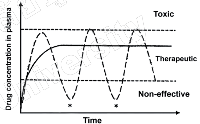
ภาพที่ 2 การเปลี่ยนแปลงความเข้มข้นของยาในร่างกายผู้ป่วยที่เวลาต่างๆ เมื่อมีการให้ยาด้วยระบบนำส่งยาแบบเดิม (---) กับแบบควบคุมการปลดปล่อย (—) (Edlund & Albertsson, 2002)
